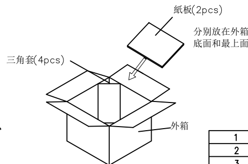
④ 产品入外箱示意图
